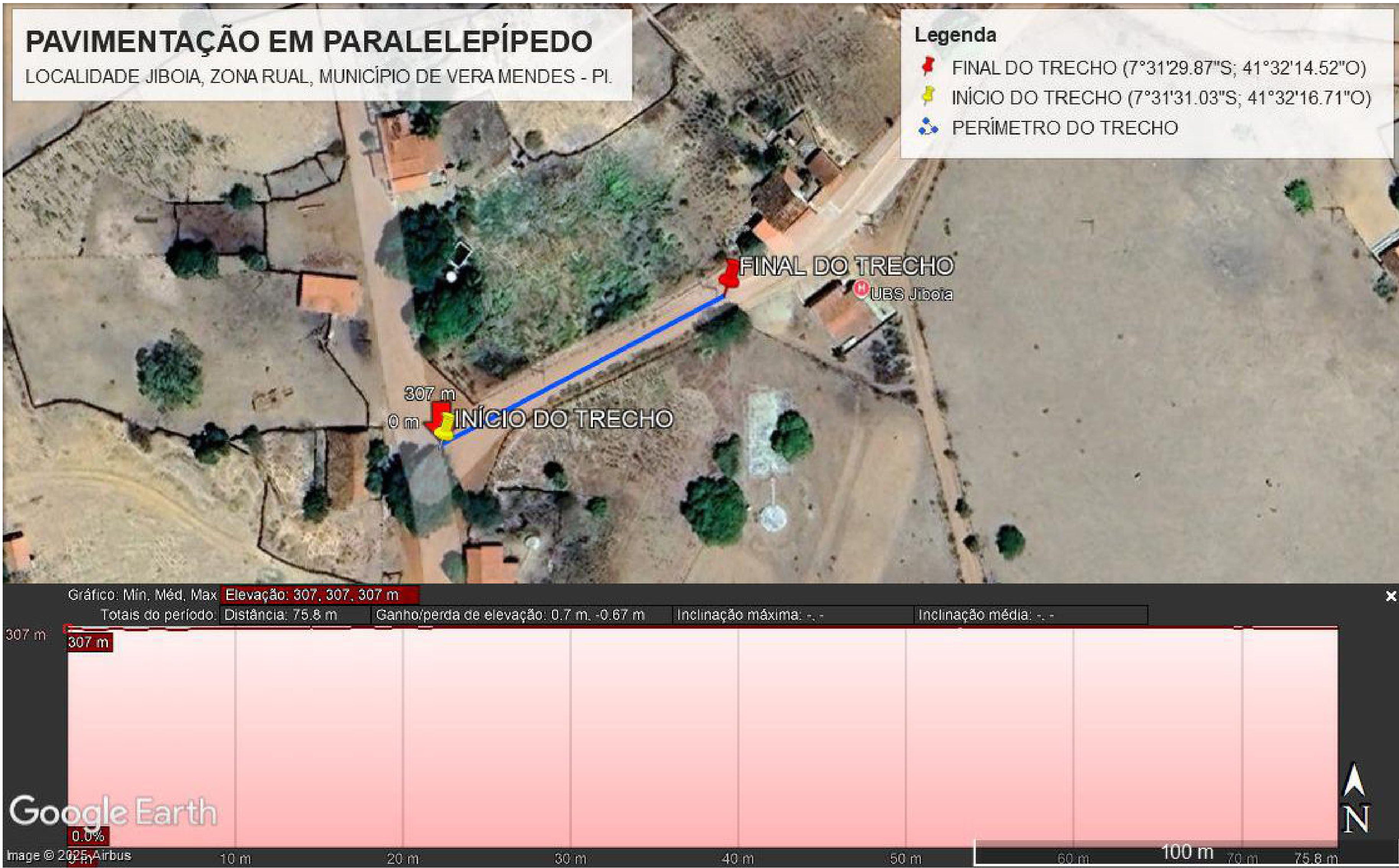
PLANTA ILUMINADA E PERFIL DE ELEVAÇÃO
