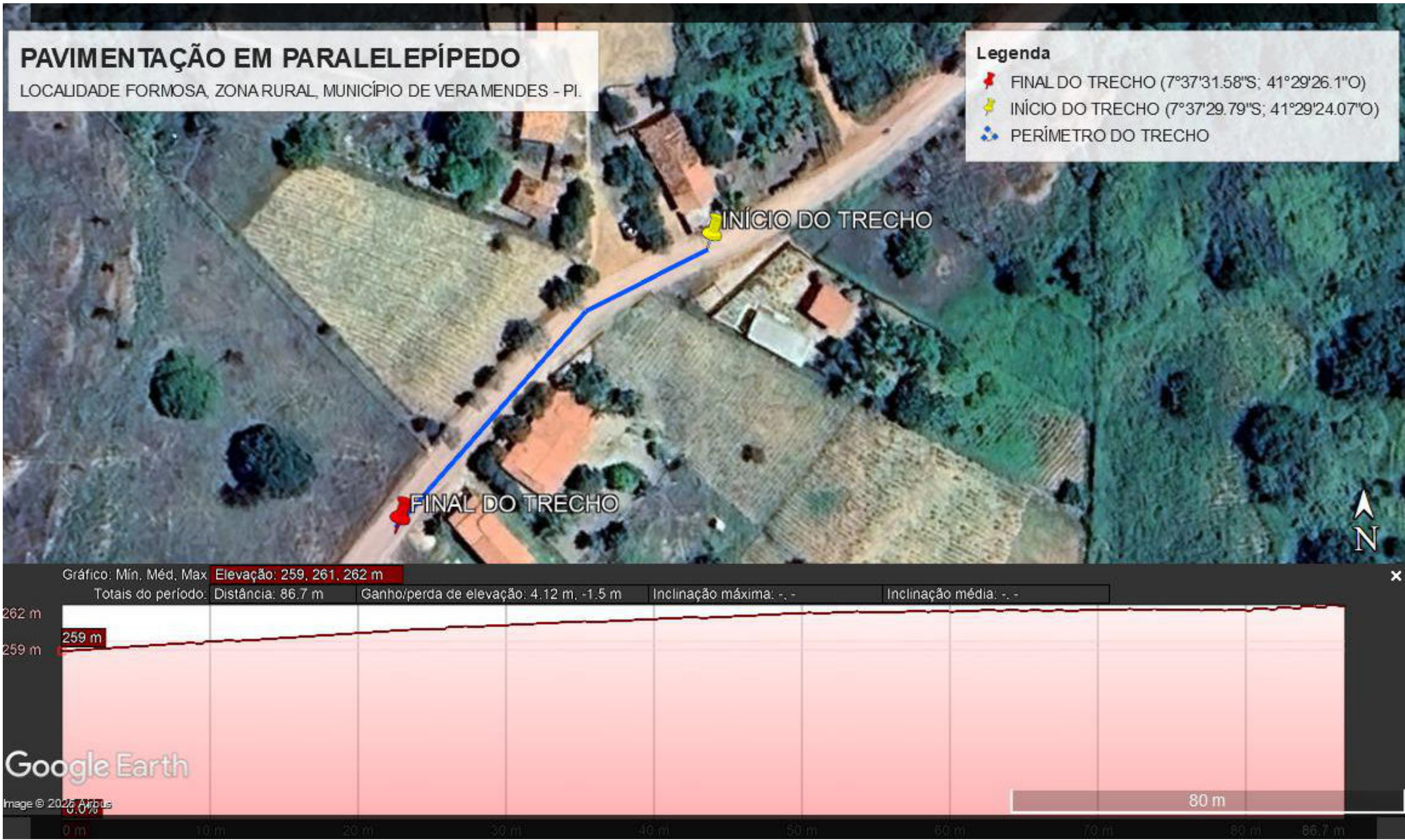
PLANTA ILUMINADA E PERFIL DE ELEVAÇÃO
